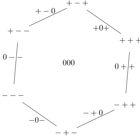
FIGURE 2.4. (Z(V), + + +) and G_2(Z(V), + + +) for example 2.25
